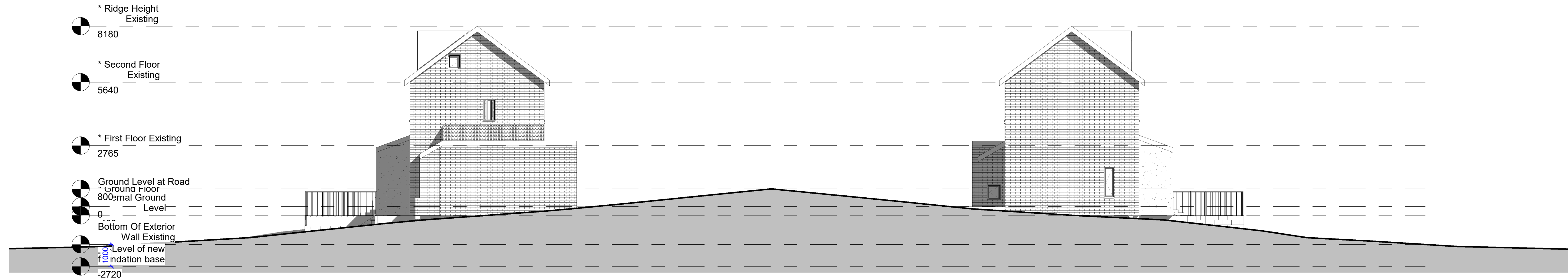
East 1 : 100
