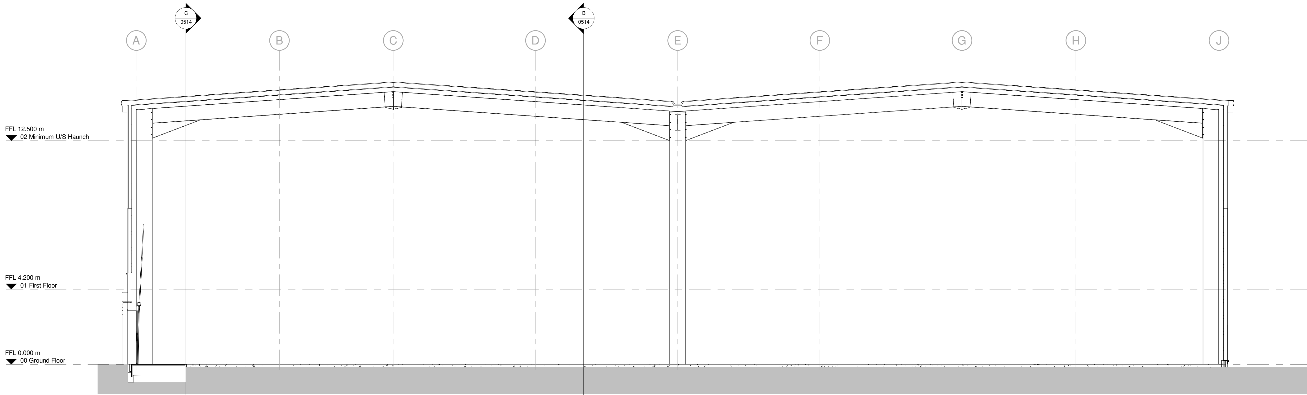
Section A-A
