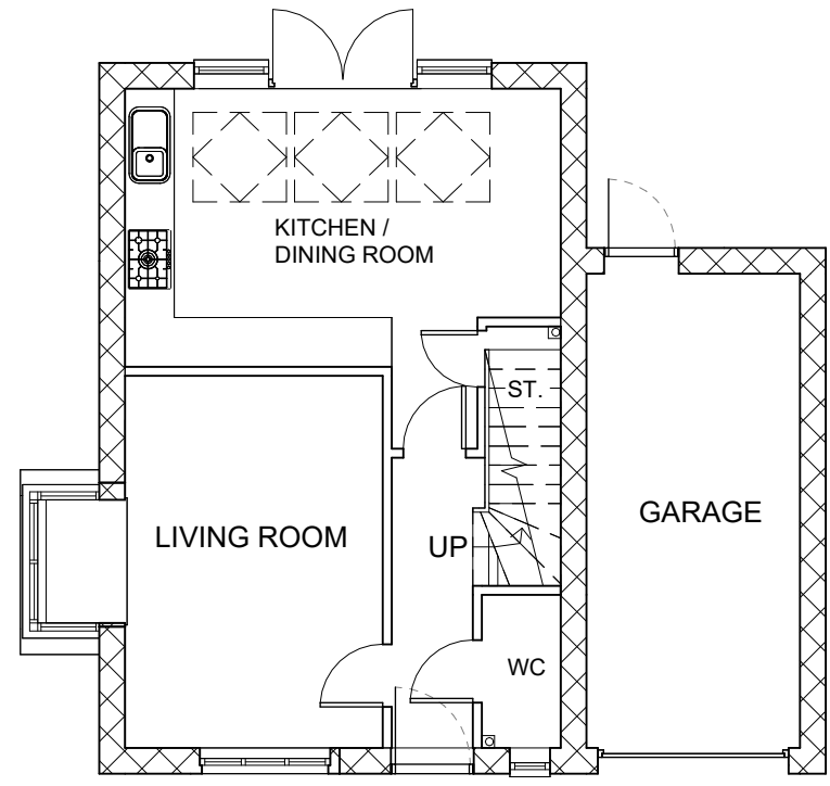
1 Existing GF 1 : 100
