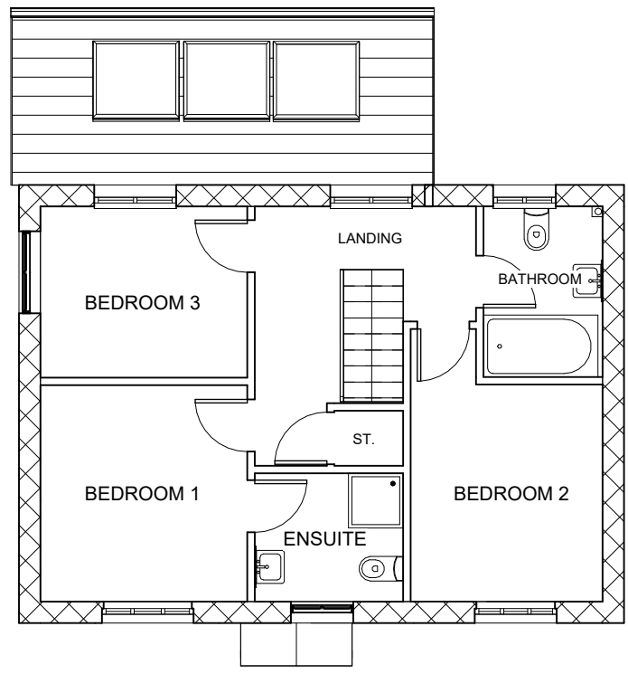
2 Existing 1F 1 : 100
