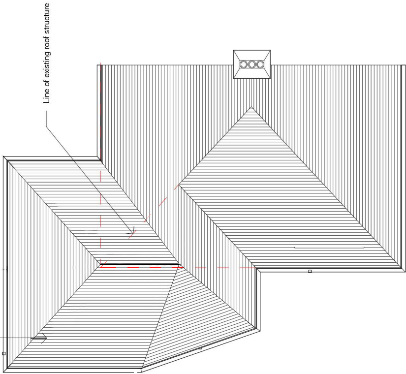
Roof Plan 1 : 100
