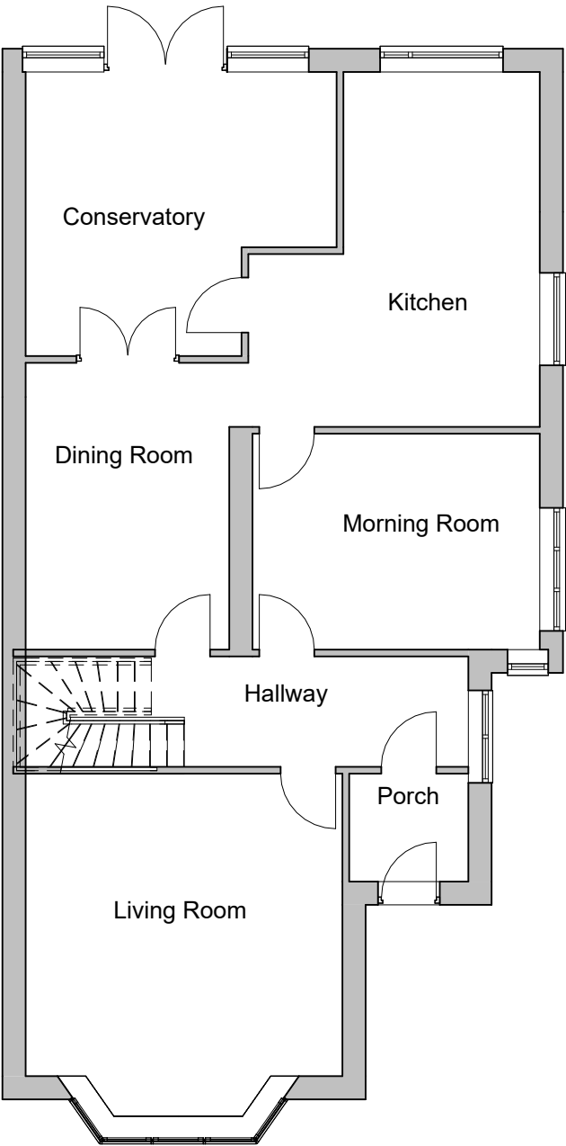
00_Ground Floor 1 : 100
