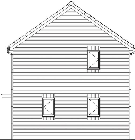
R.H. Side Elevation
