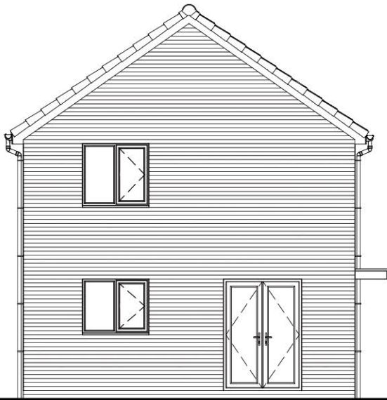
L.H. Side Elevation
