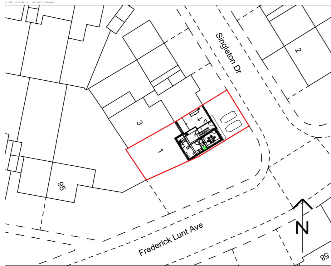
SITE PLAN 1:500
