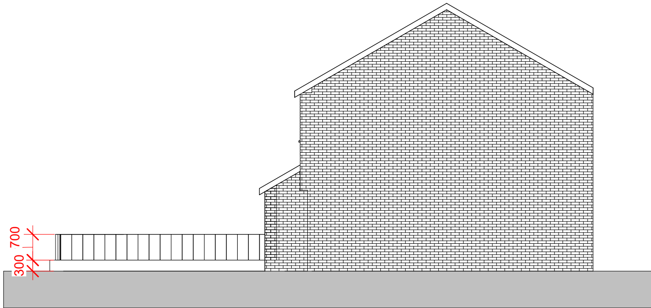
East 1 : 100
