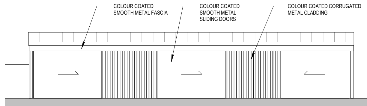
ELEVATION A
