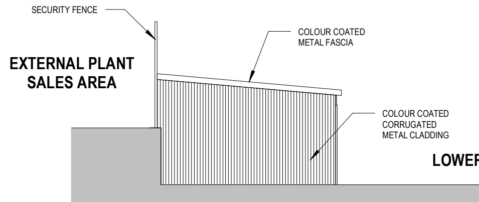
ELEVATION B
