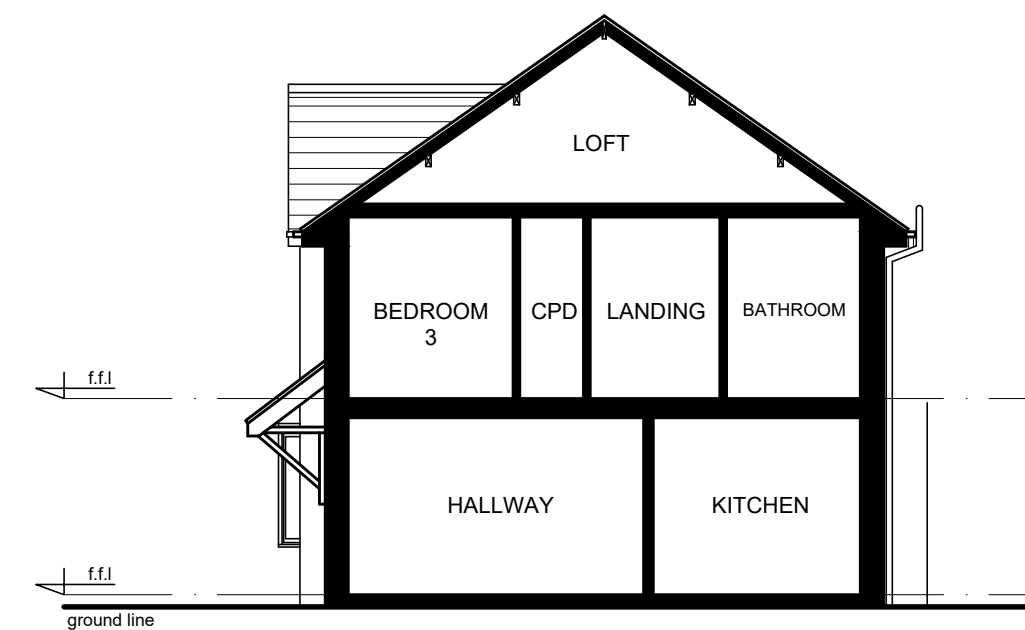
RIGHT ELEVATION
