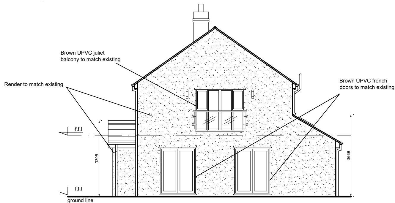
RIGHT ELEVATION
