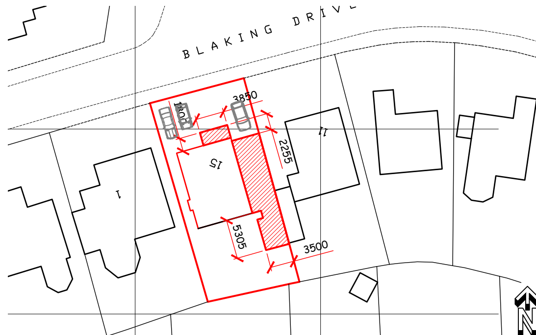
SITE PLAN 1:500
