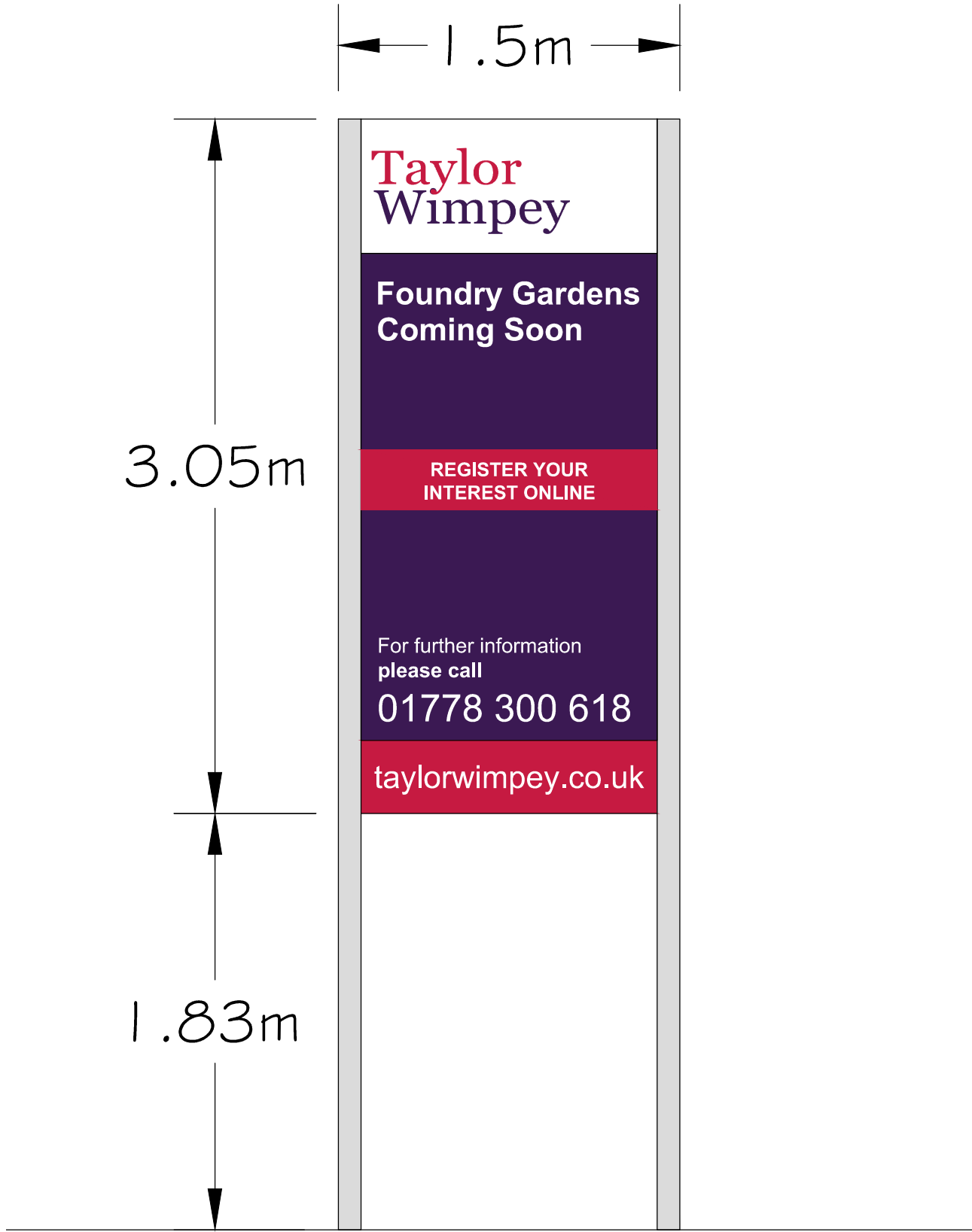
V-Stack Sign (Scale 1:25)
