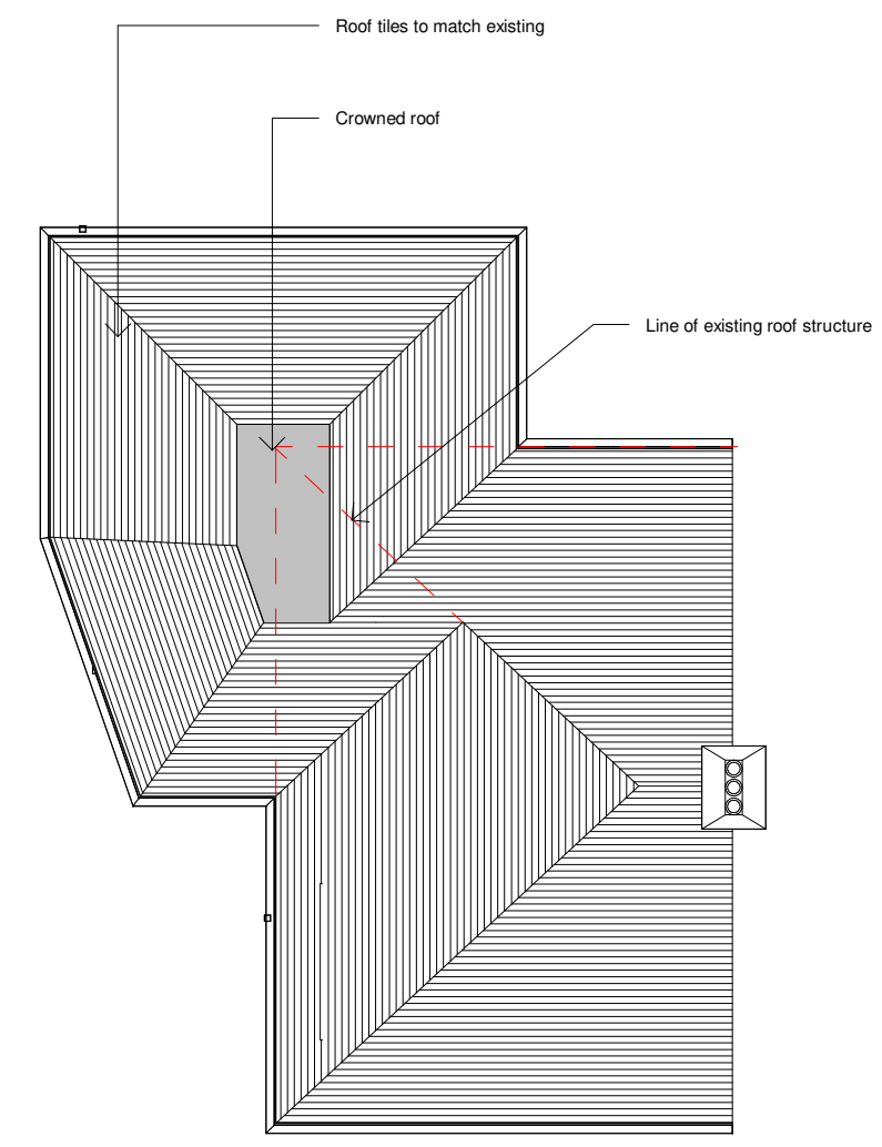
Roof Plan 1 : 100
