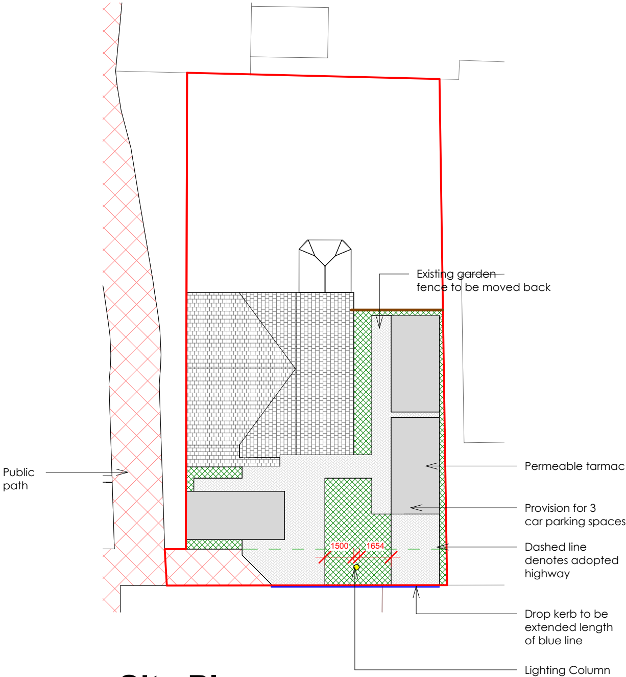
Site Plan 1 : 200
