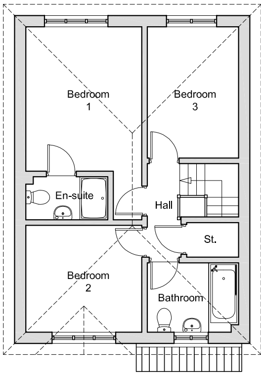
Existing 1/F Plan 1:100
