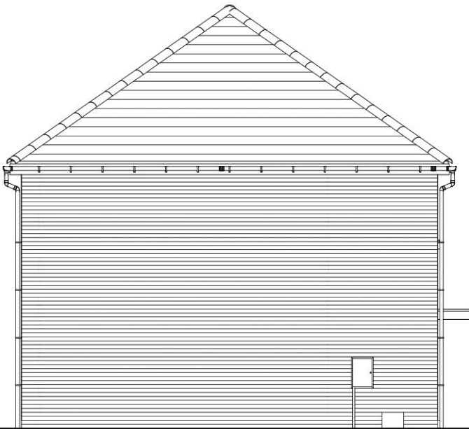
L.H. / R.H. Side Elevation
