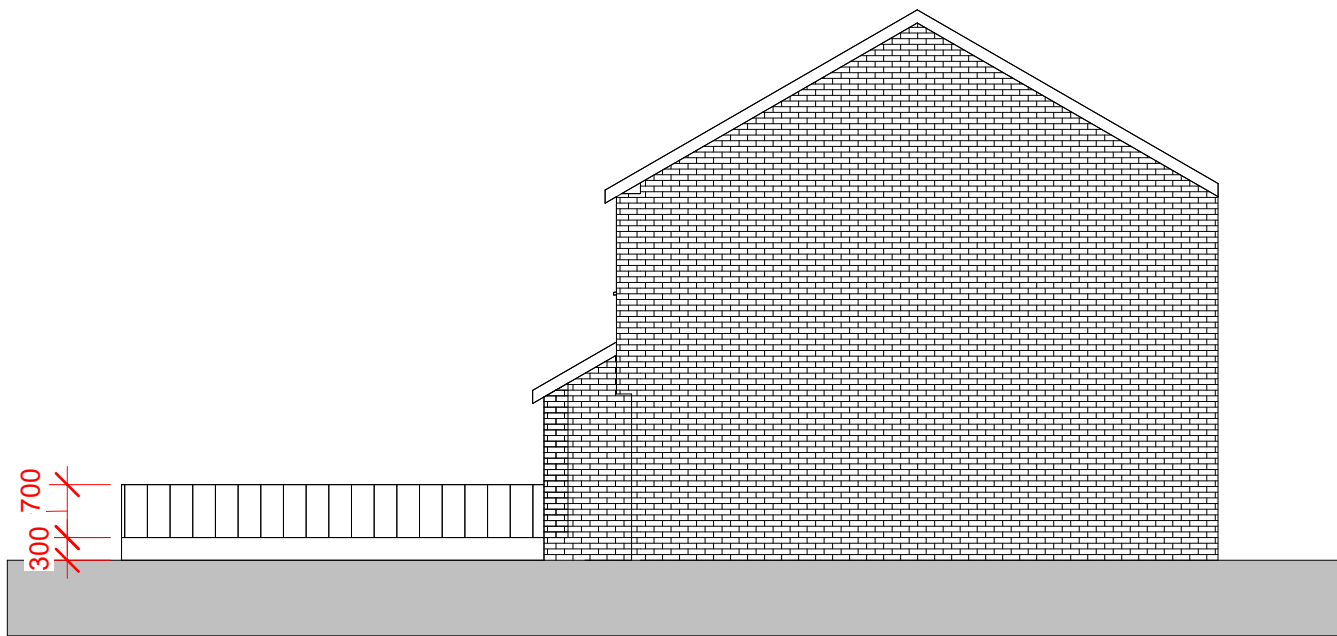
East 1 : 100
