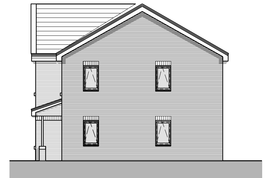
South Elevation (D)
