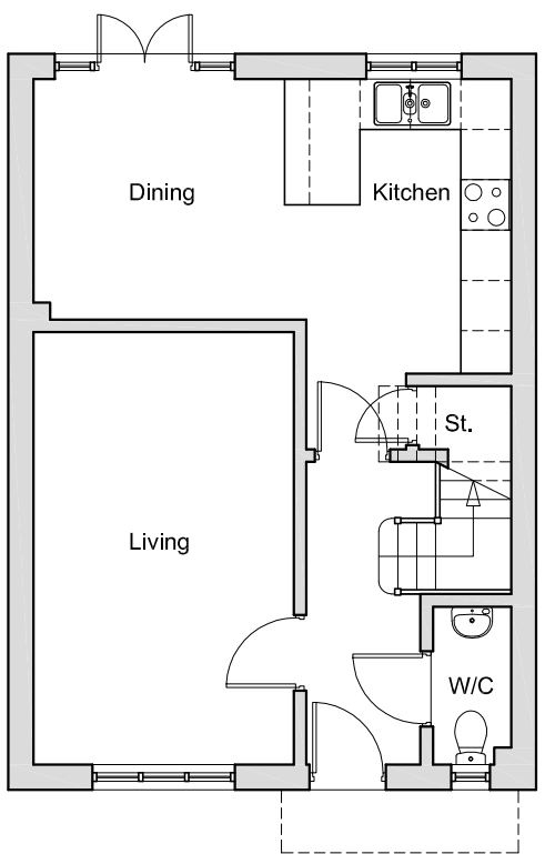
Existing G/F Plan 1:100
