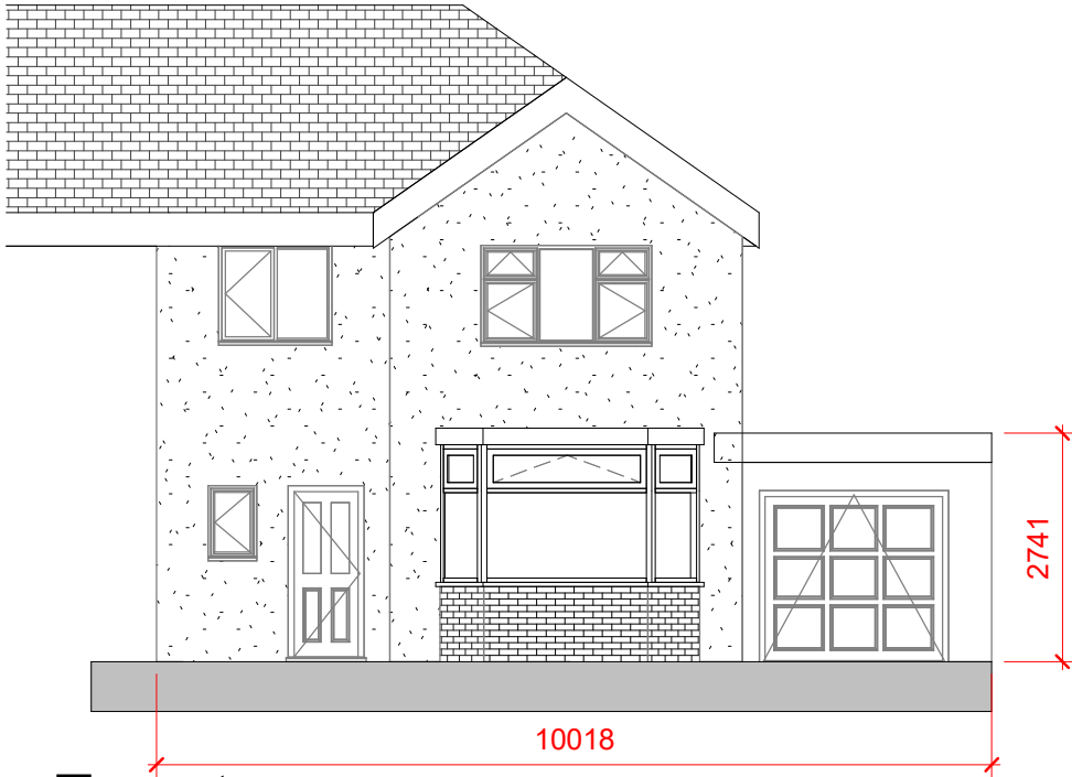
Front 1 : 100
