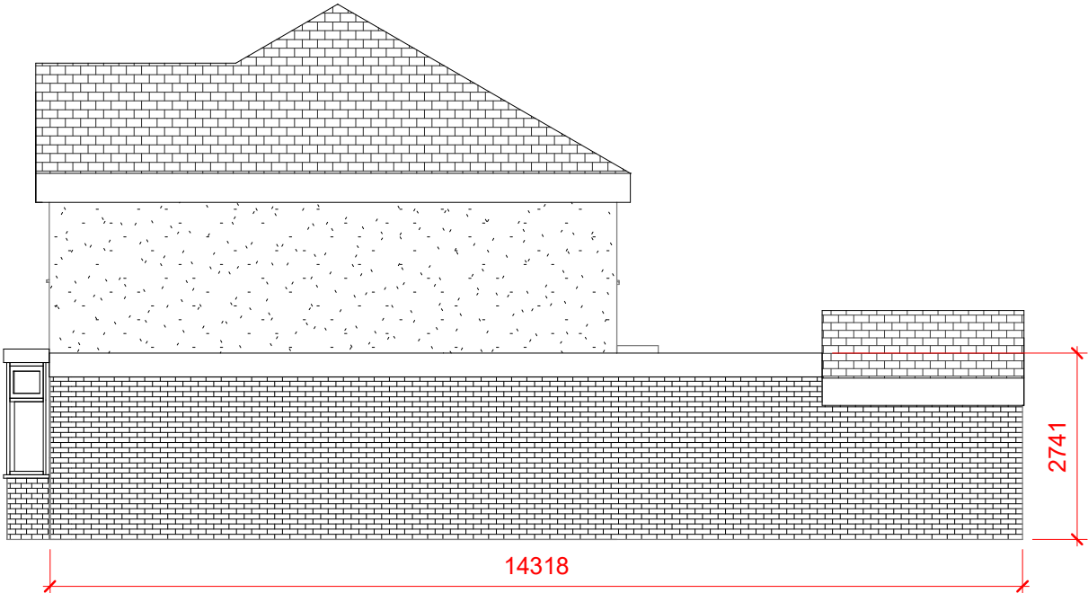
East 1 : 100
