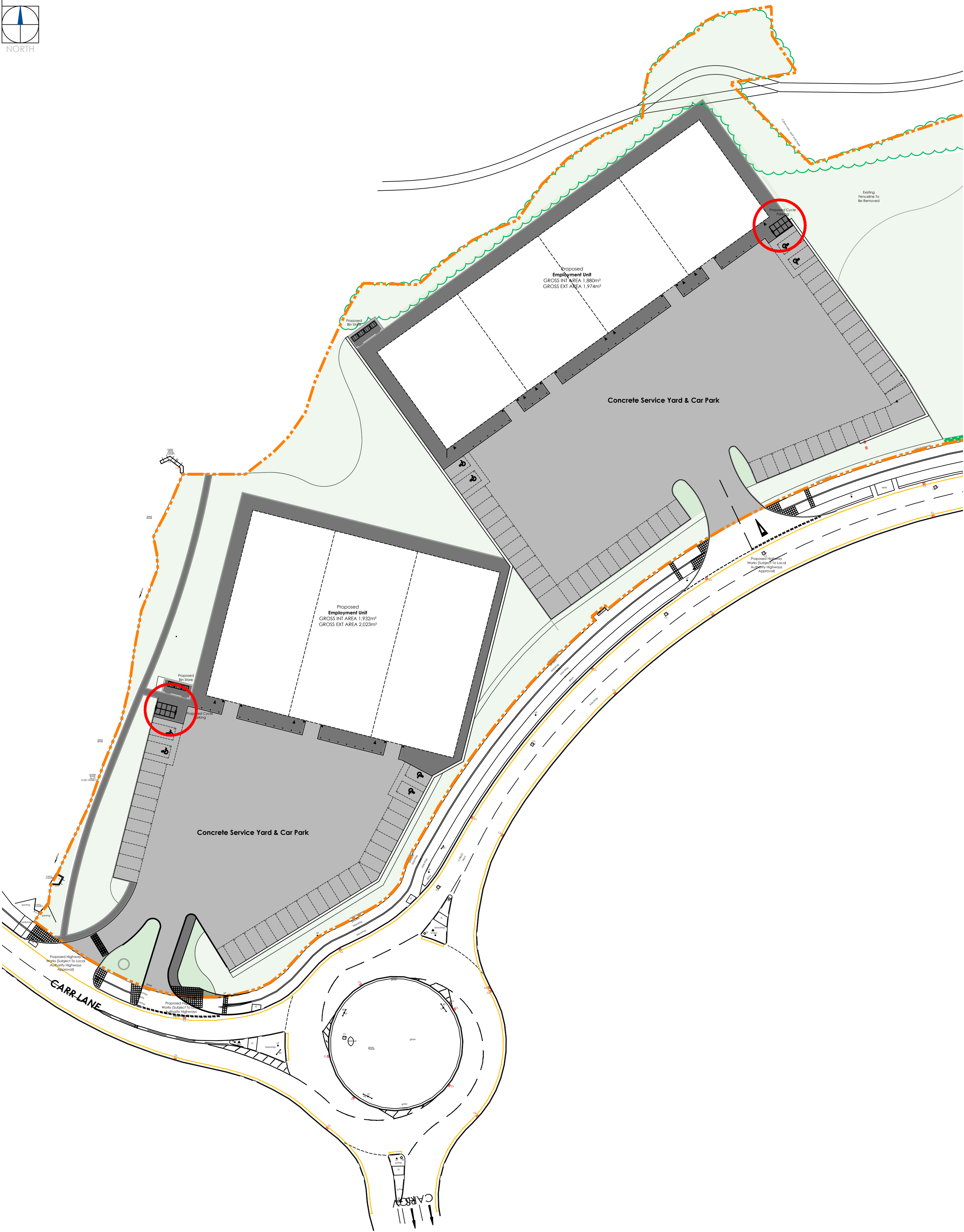
Site Plan - 1:500
