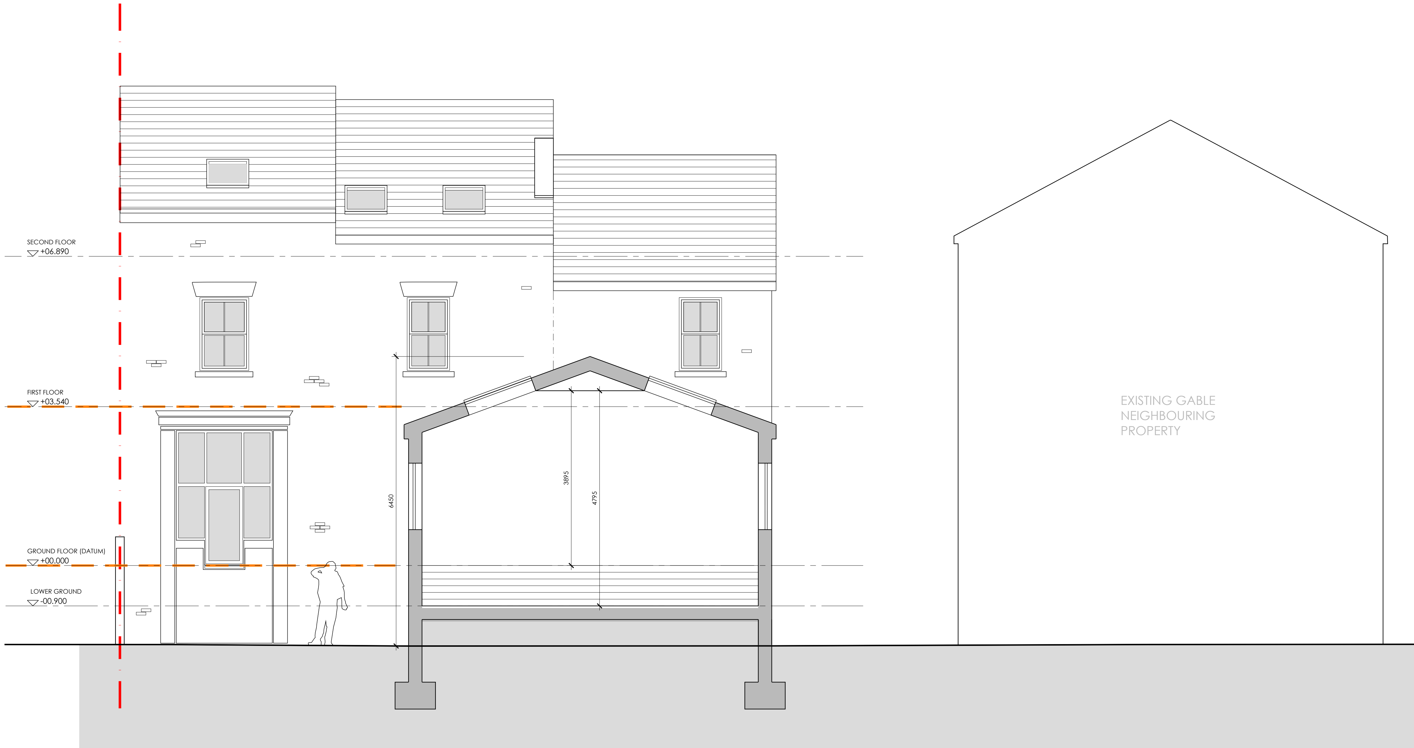
1 SECTION A-A 1:50
