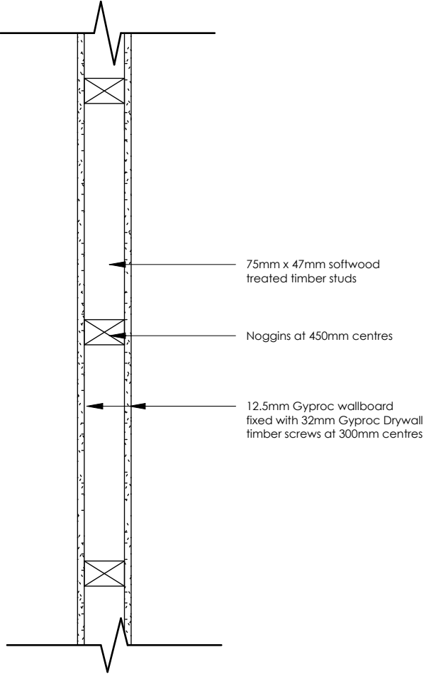
GBA-IW1 Internal Timber stud wall
