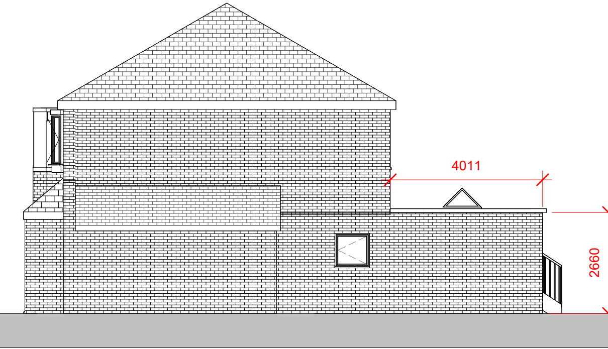
East 1 : 100
