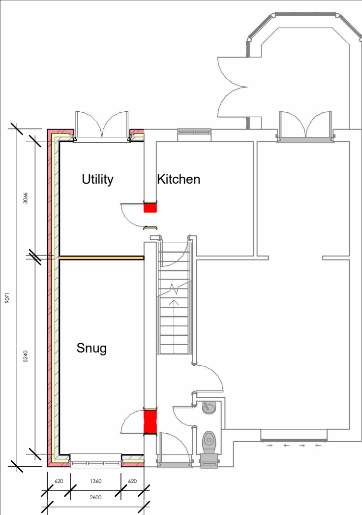
00_Ground Floor 1 : 100
