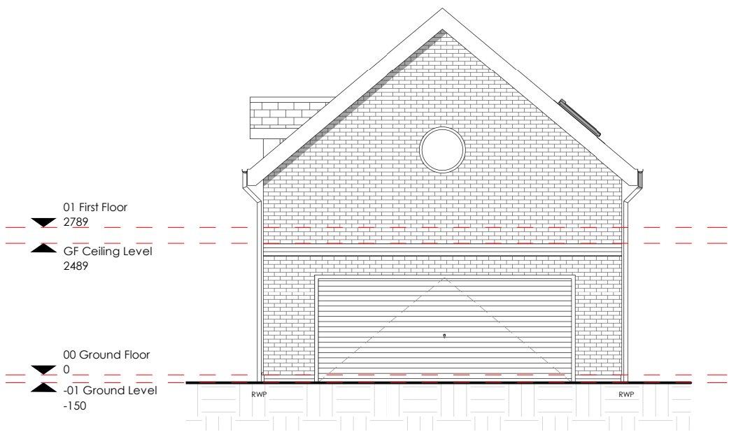
Elevation 1
