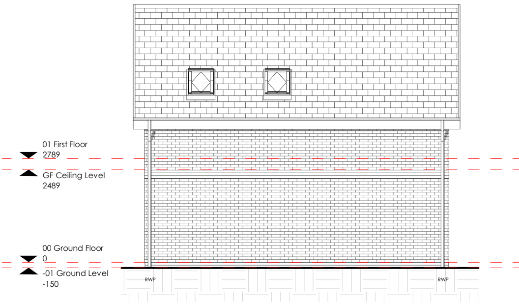
Elevation 4
