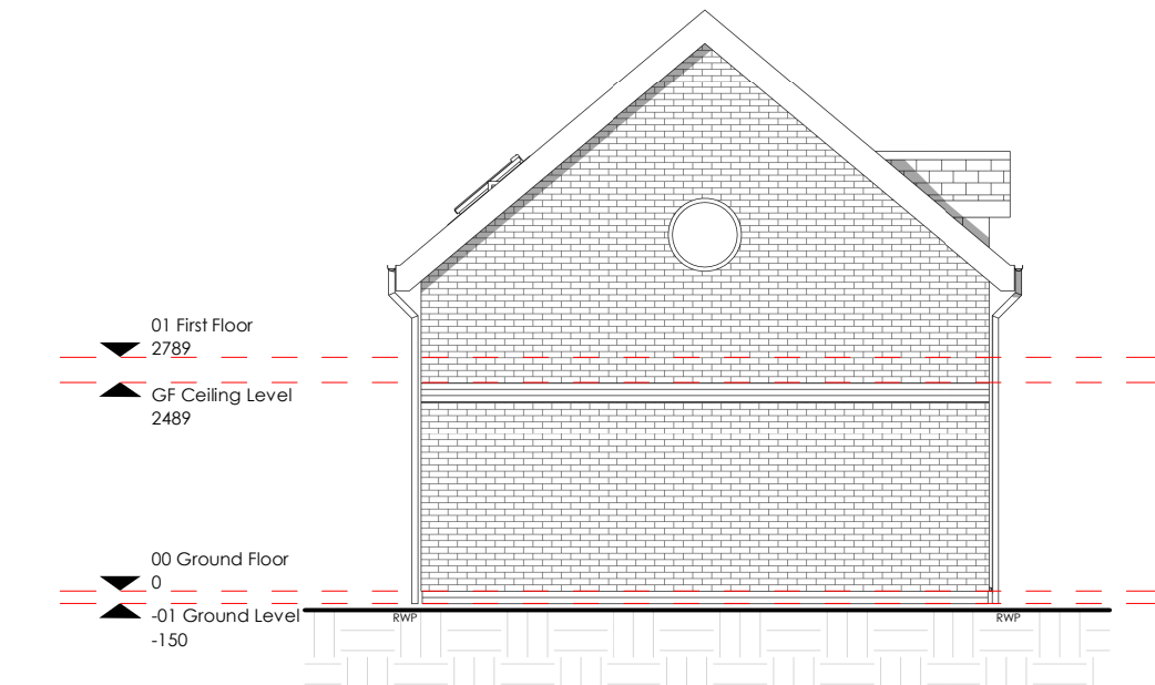
Elevation 3
