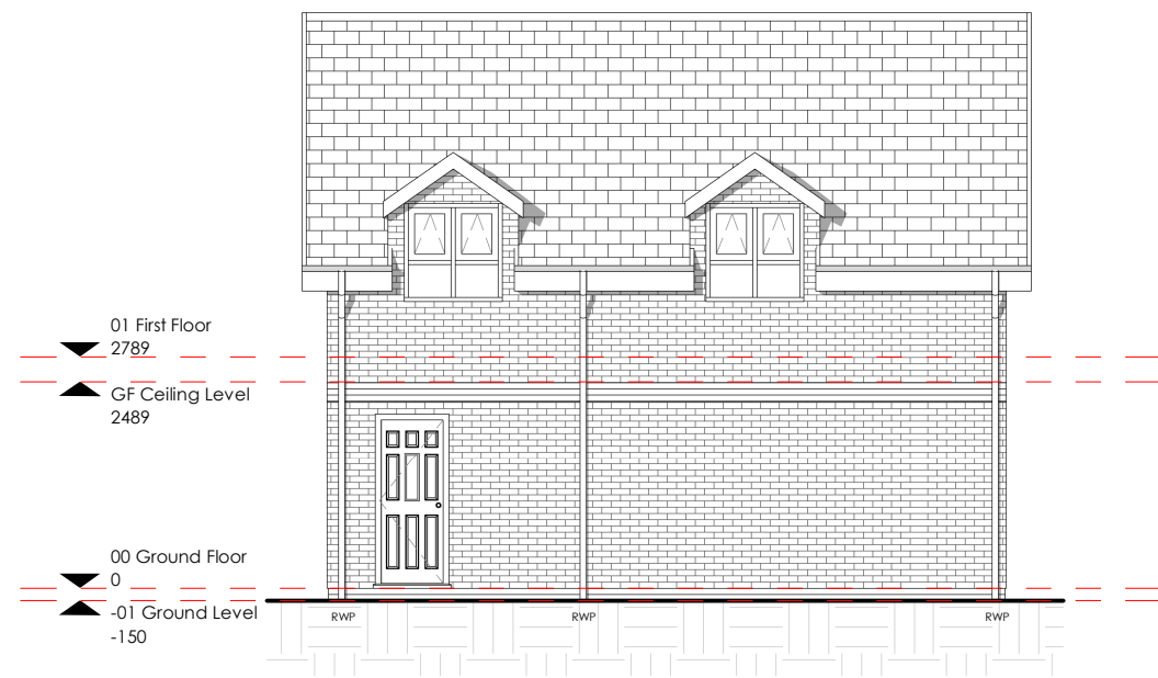
Elevation 2
