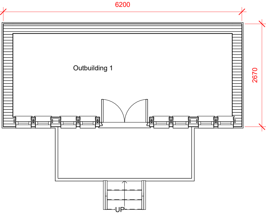
00_Ground Floor OB 1 1 : 50
