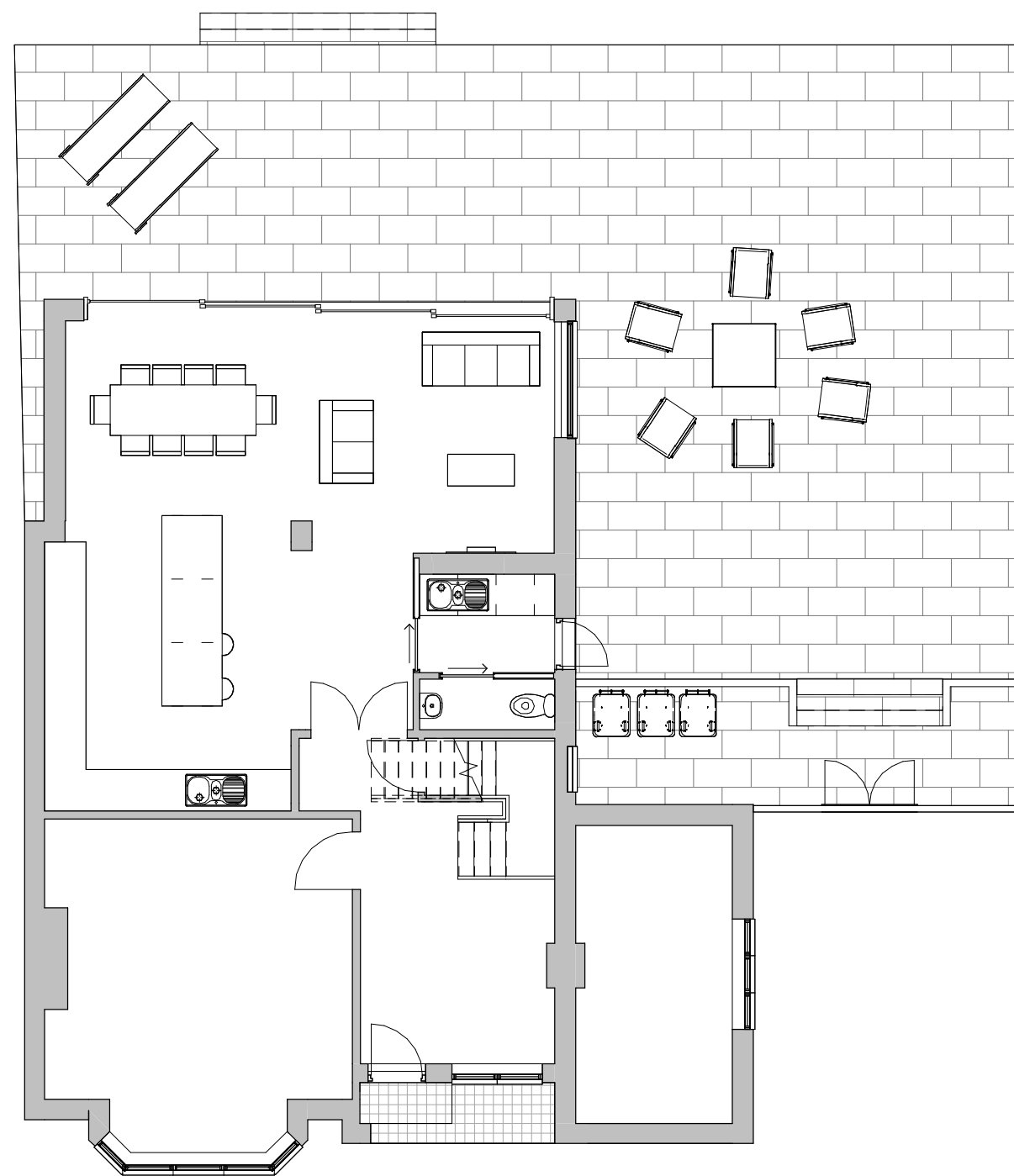
0 Level 0 1 : 100
