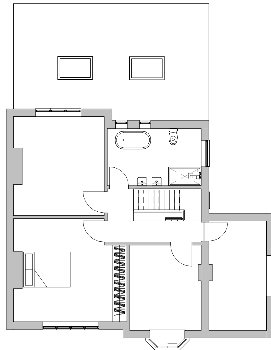
1 Level 1 1 : 100
