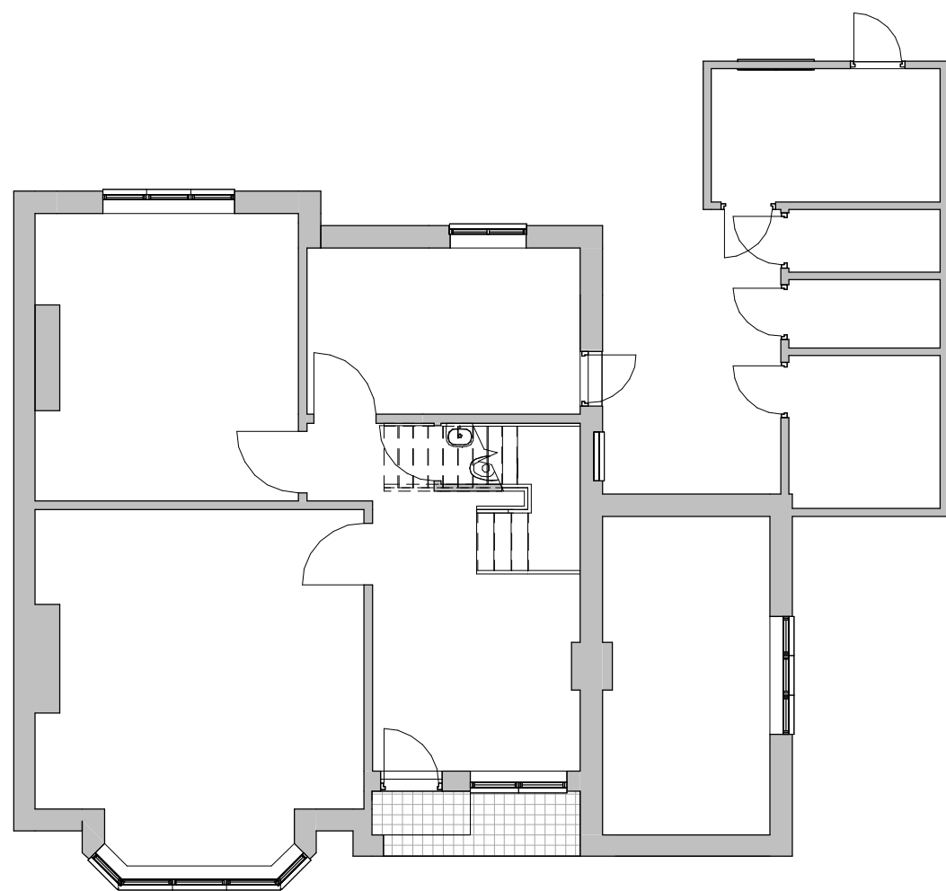
0 Level 0 1 : 100
