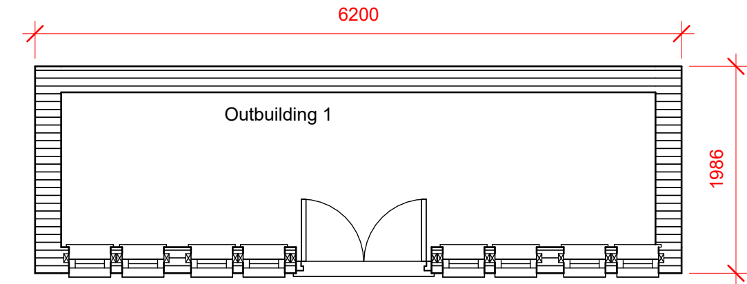
00_Ground Floor OB 1 1 : 50
