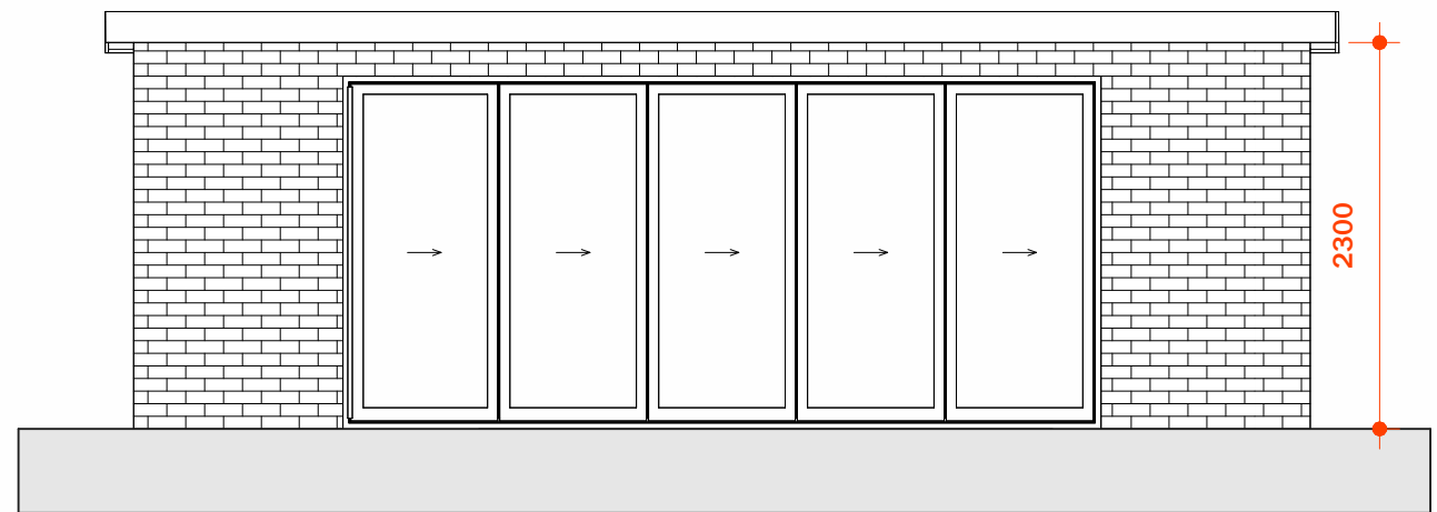
2 Rear Elevation SCALE: 1 : 50
