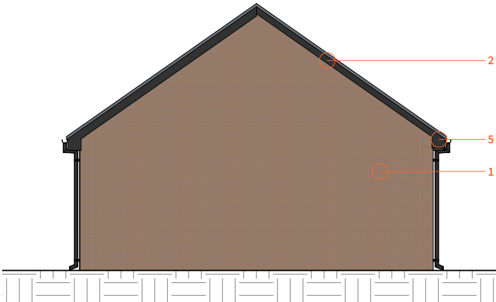
RHS Elevation
