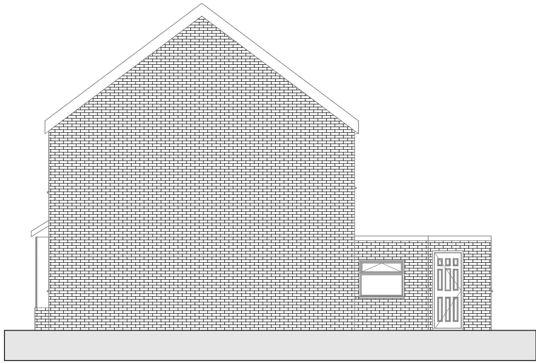
5 Existing East SCALE: 1 : 100
