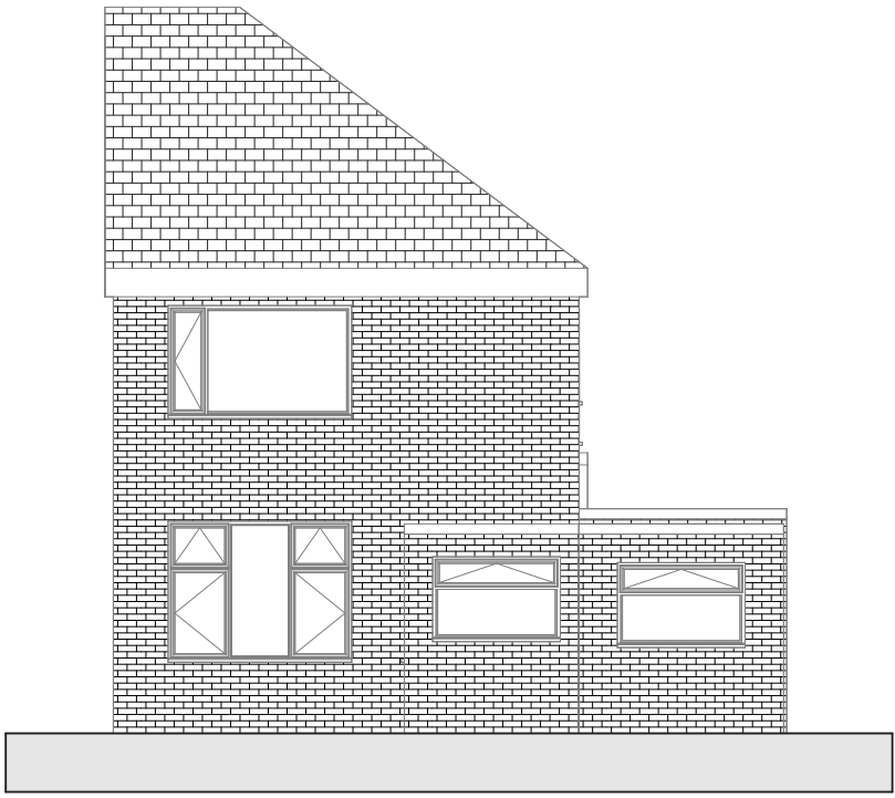
2 EXISTING REAR SCALE: 1 : 100
