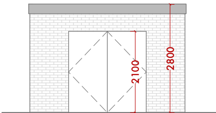
02a Elevation
