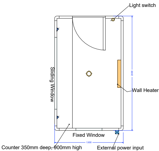
KIOSK FLOOR PLAN
