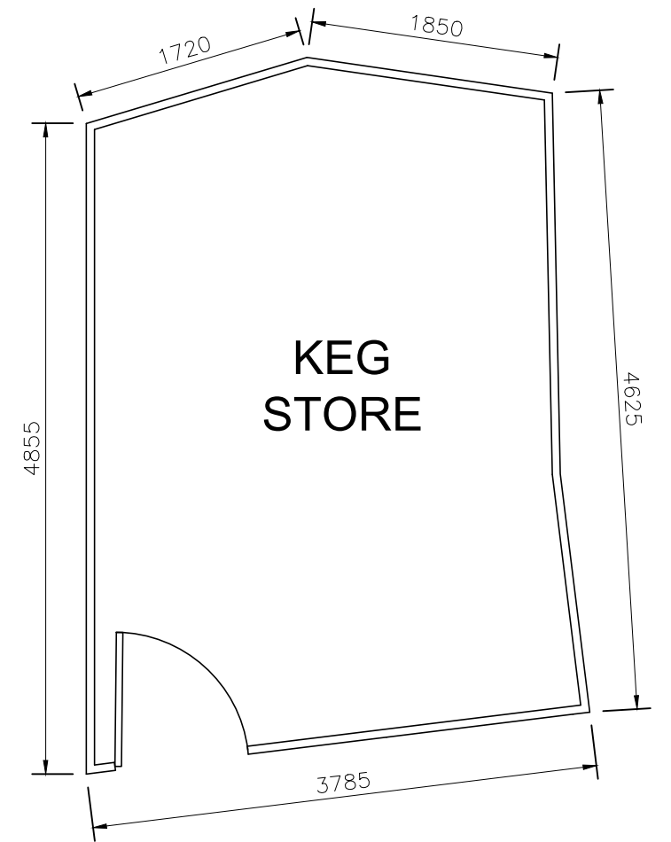
KEG STORE: PLAN
