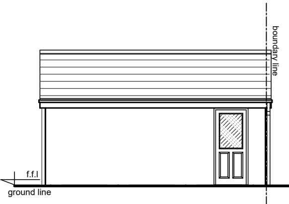
RIGHT ELEVATION
