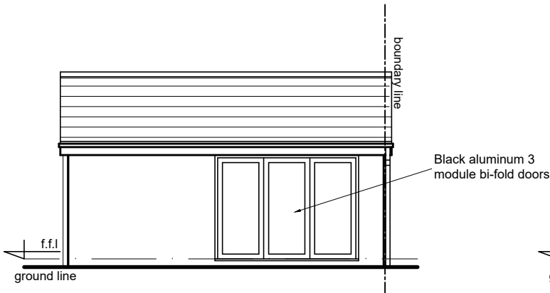
RIGHT ELEVATION
