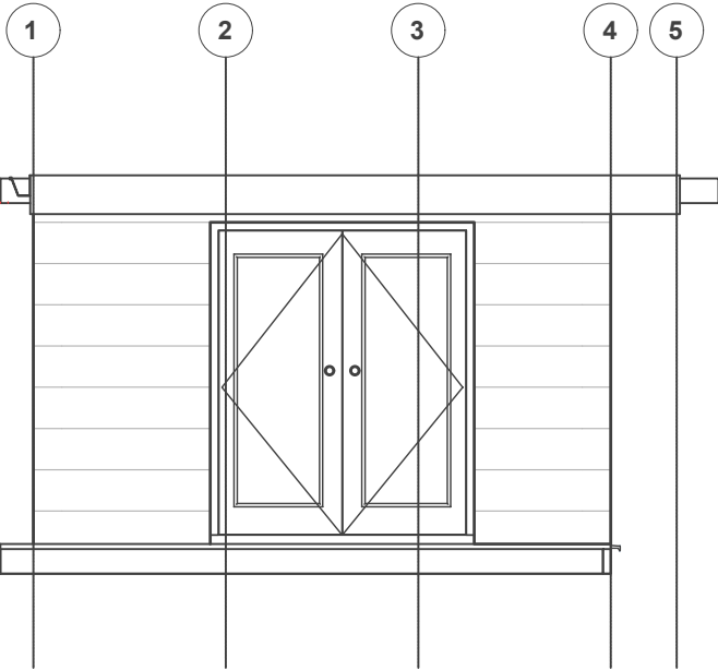
ELEVATION C LEFT 1:50
