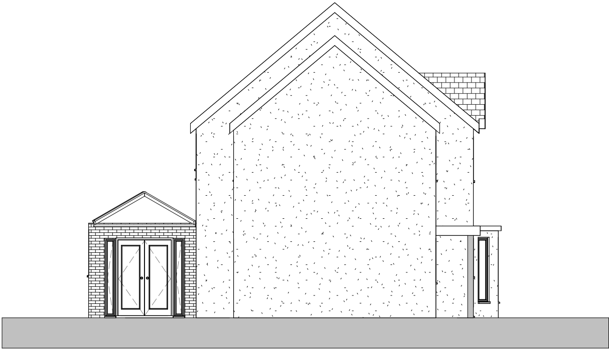
West 1 : 100
