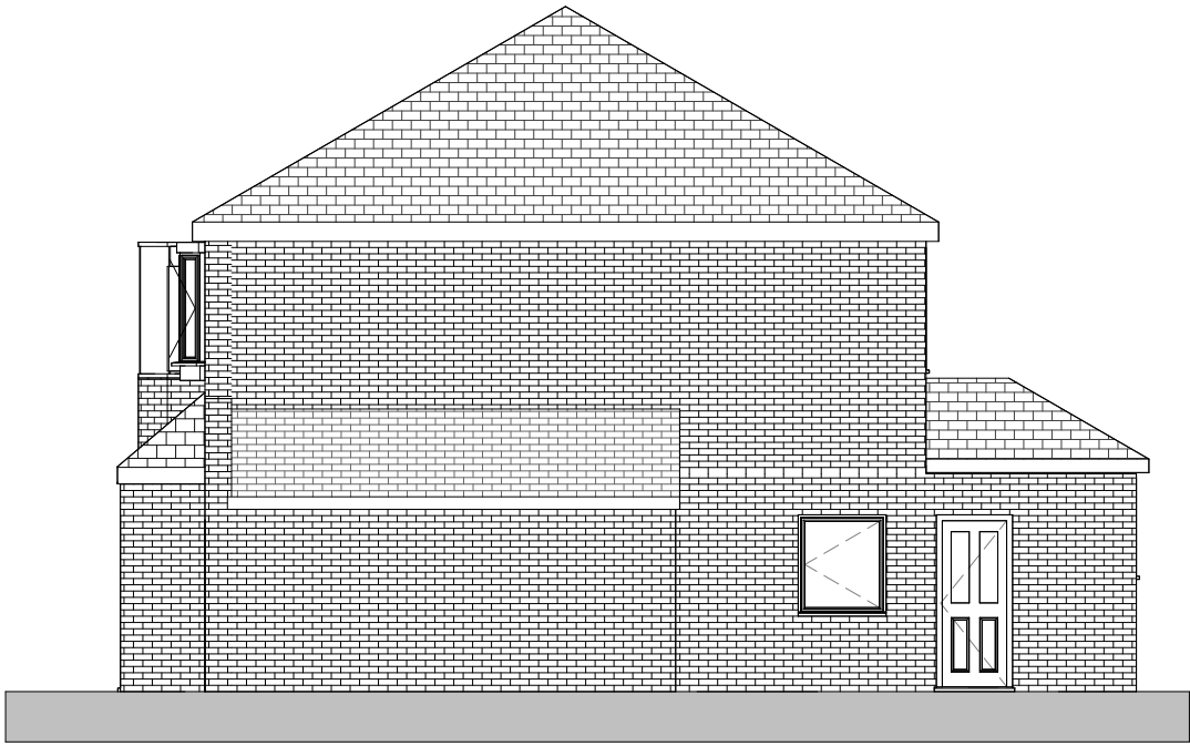
East 1 : 100
