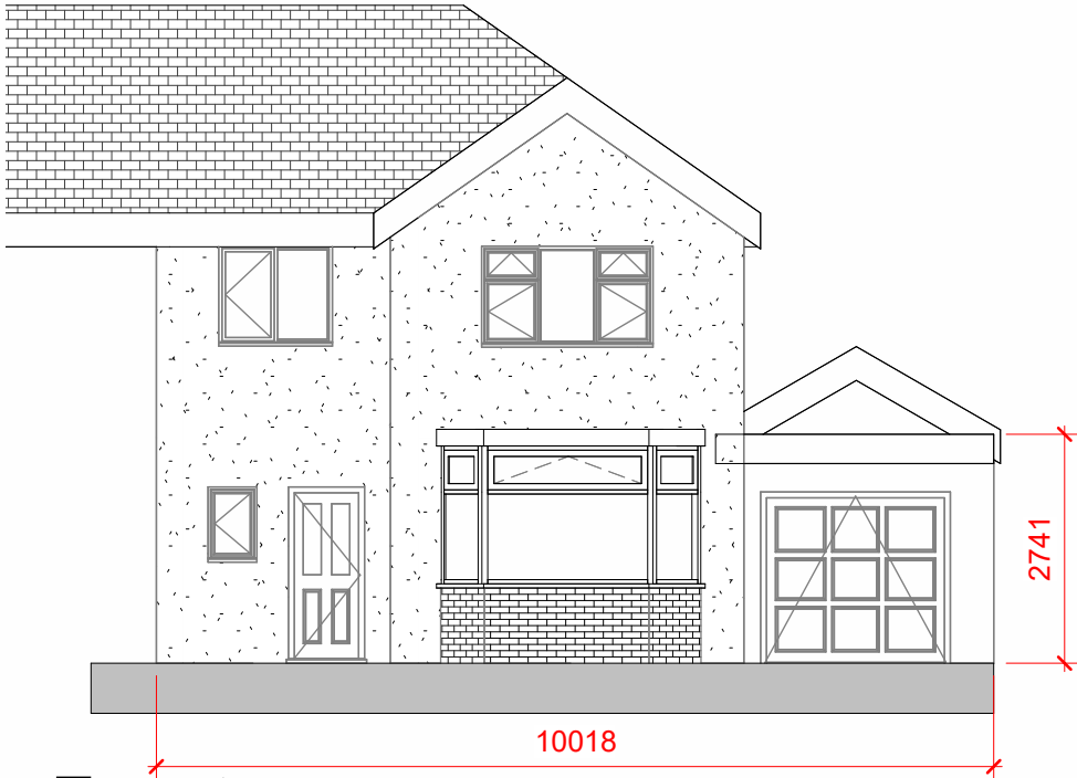
Front 1 : 100
