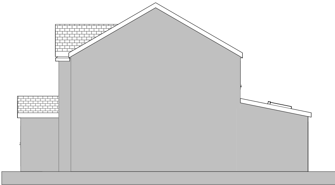
East 1 : 100
