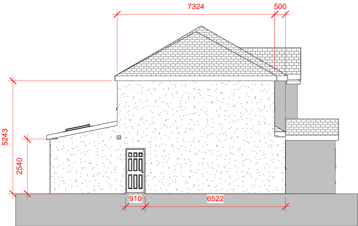
West 1 : 100
