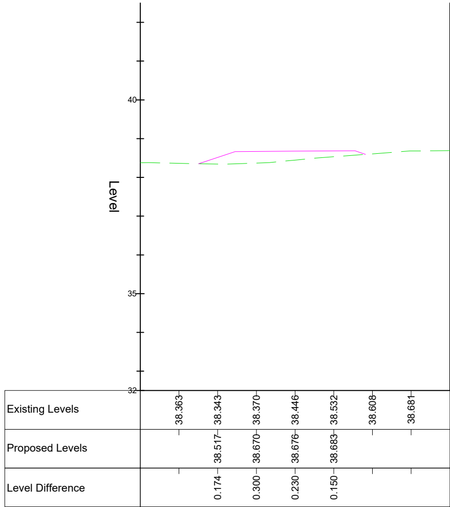
Chainage 260.000
