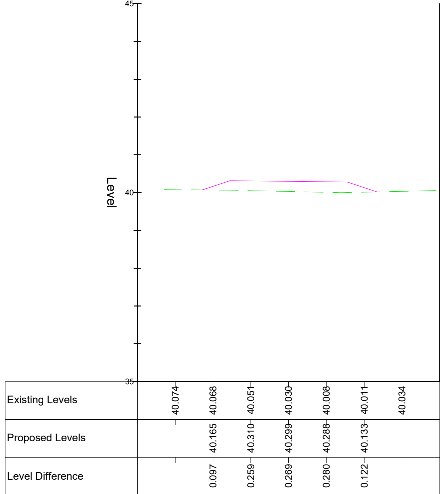
Chainage 60.000 (47)
