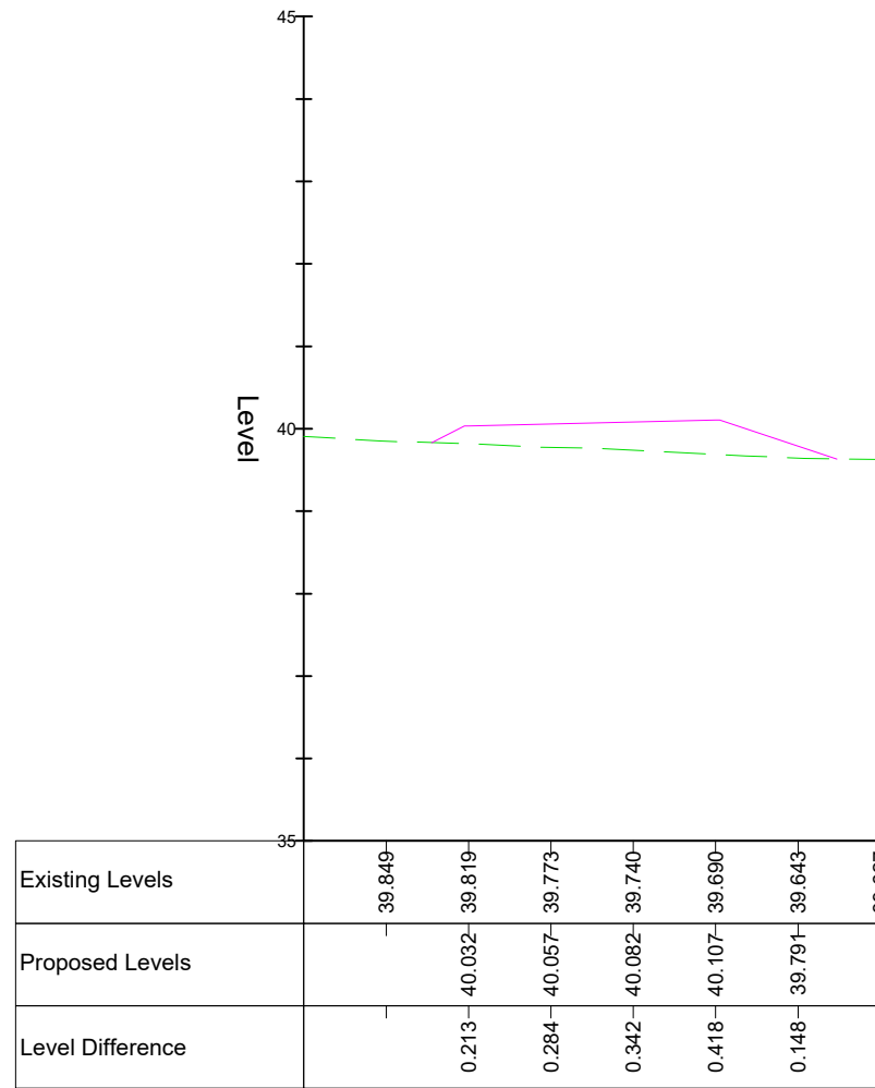
Chainage 60.000
