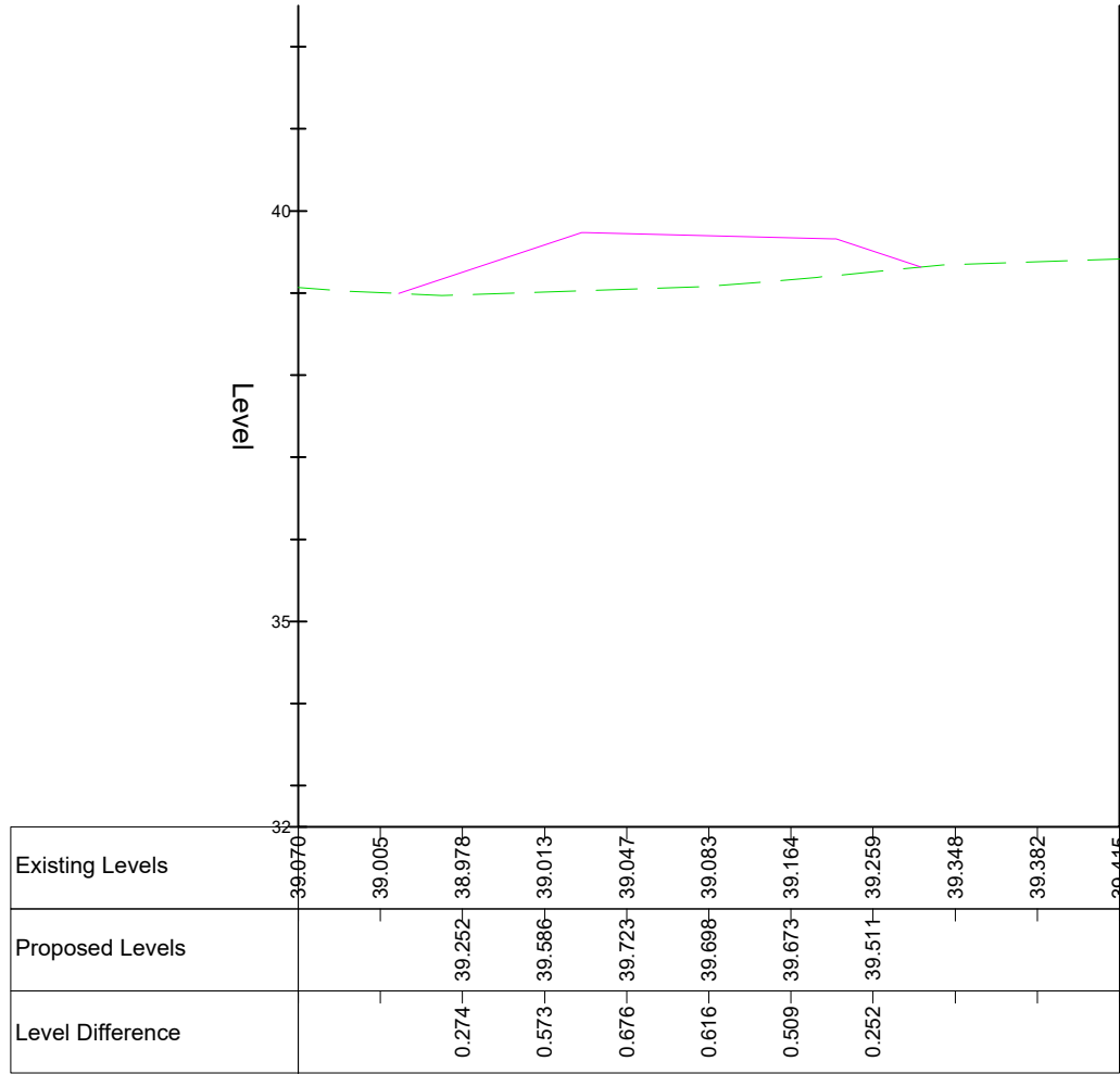
Chainage 320.000
