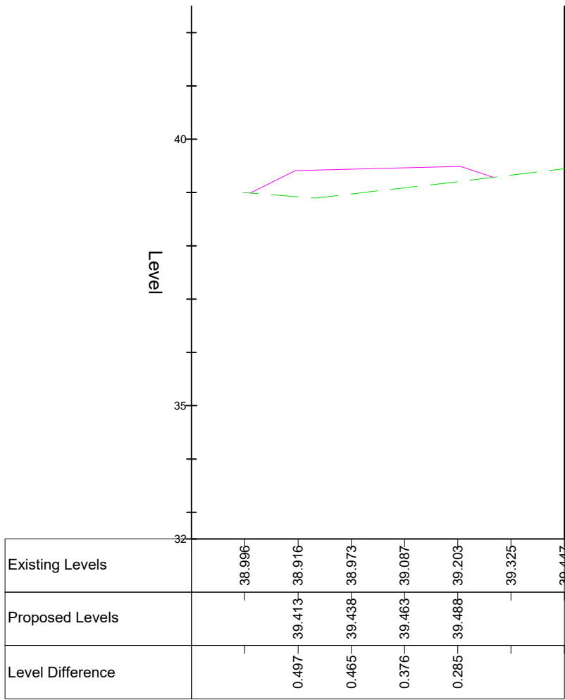
Chainage 40.000
