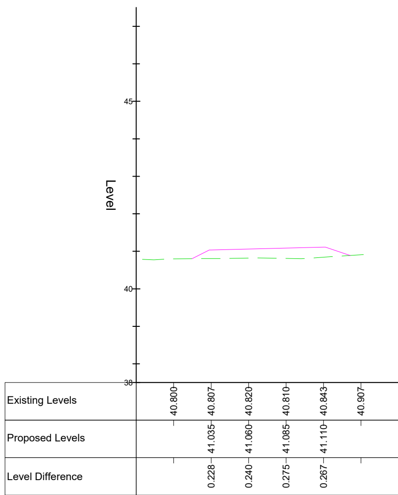
Chainage 90.000
