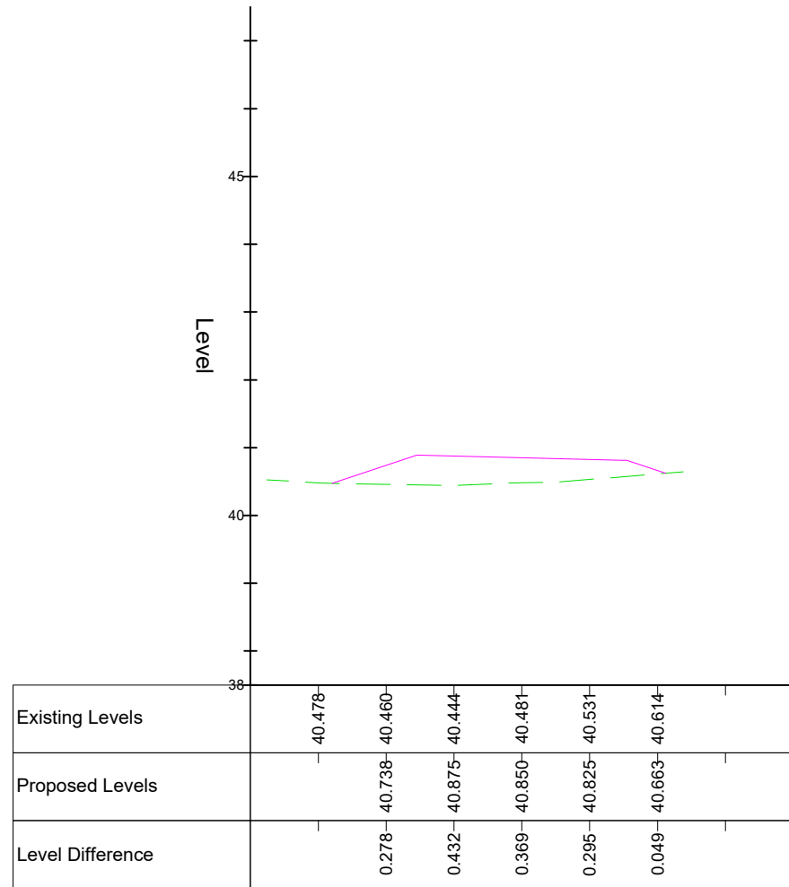
Chainage 40.000 (46)
