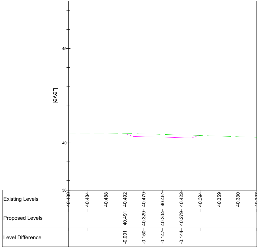
Chainage 360.000
