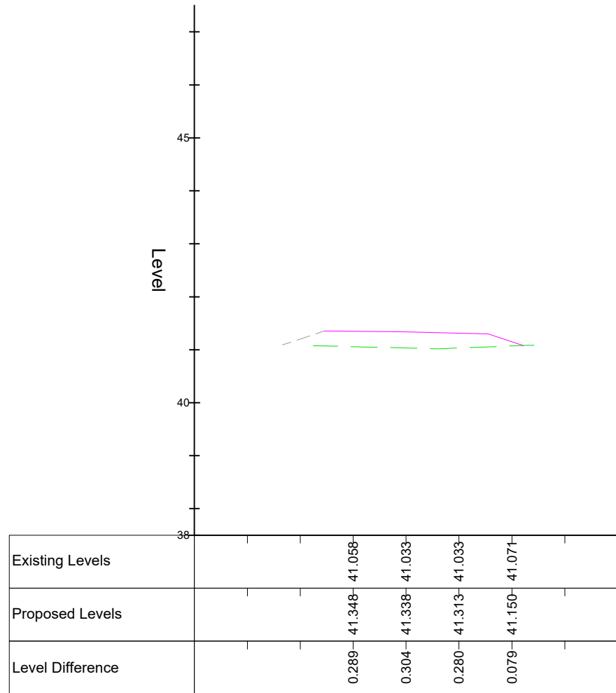
Chainage 20.000 (45)
