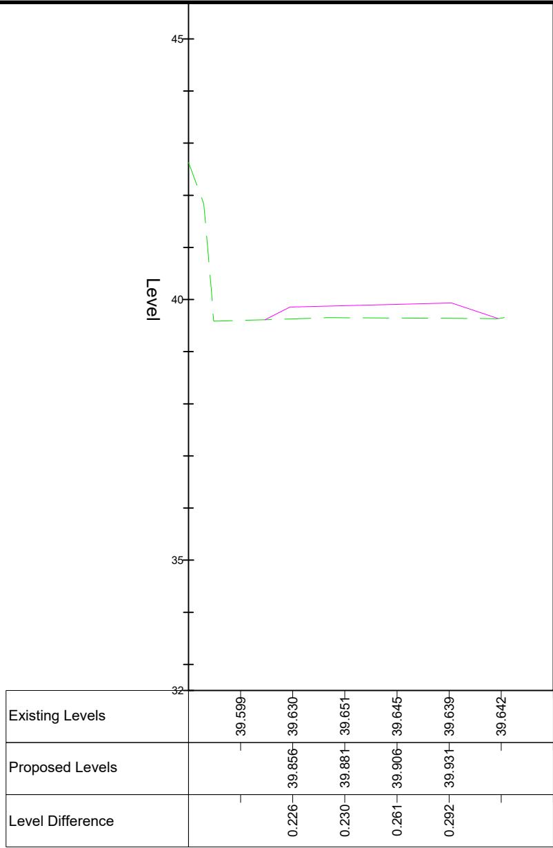
Chainage 20.000
