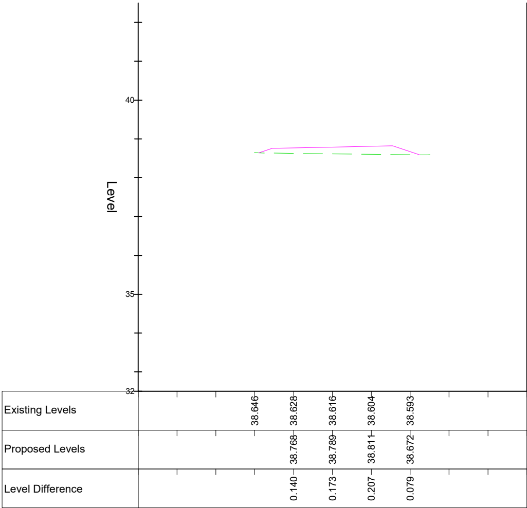
Chainage 280.000
