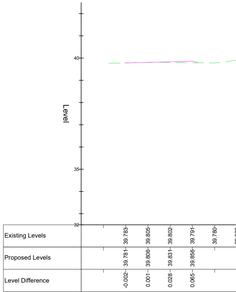
Chainage 0.000 (43)
