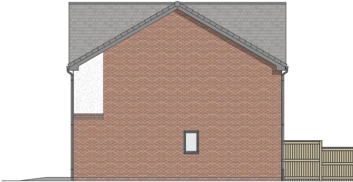
TYPE F 3B4P 86 (OPP) SIDE ELEVATION
