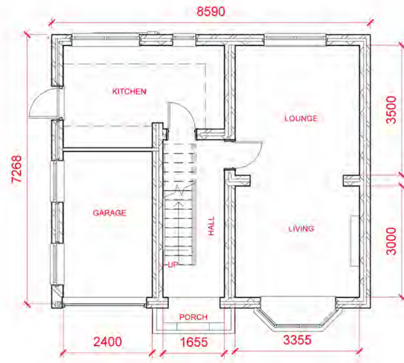
1 Level 0 1 : 100
