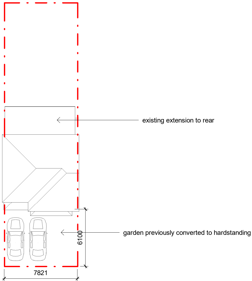
SITE PLAN 1:200
