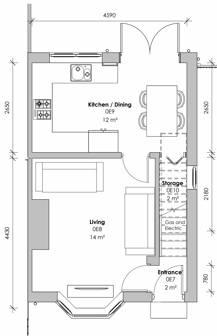
1 Level 0 - Existing 1 : 50
