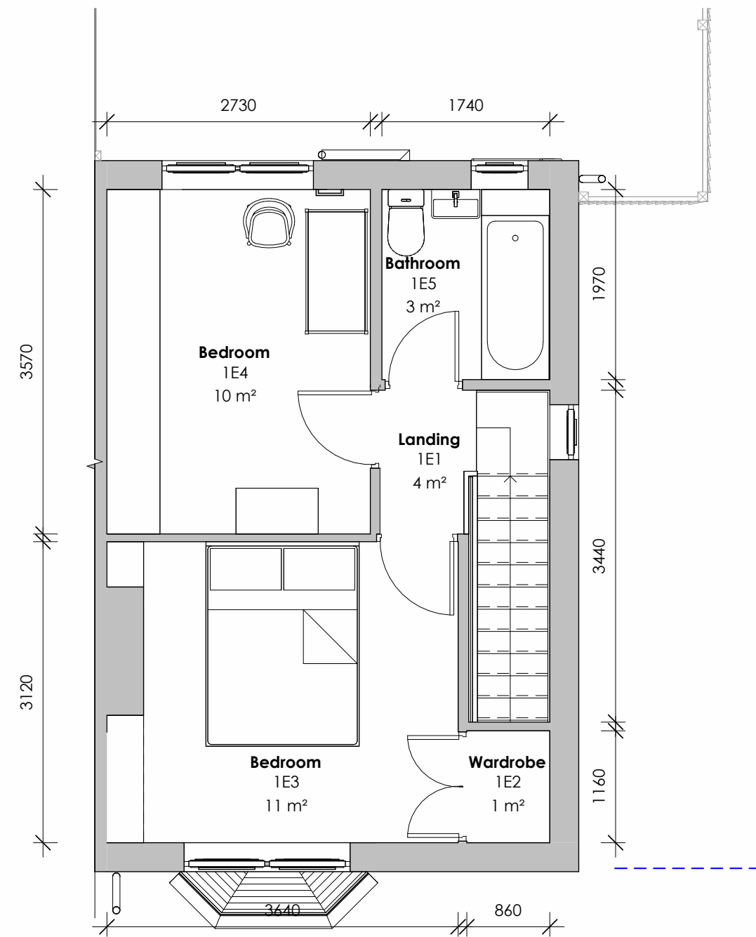
2 Level 1 - Existing 1 : 50
