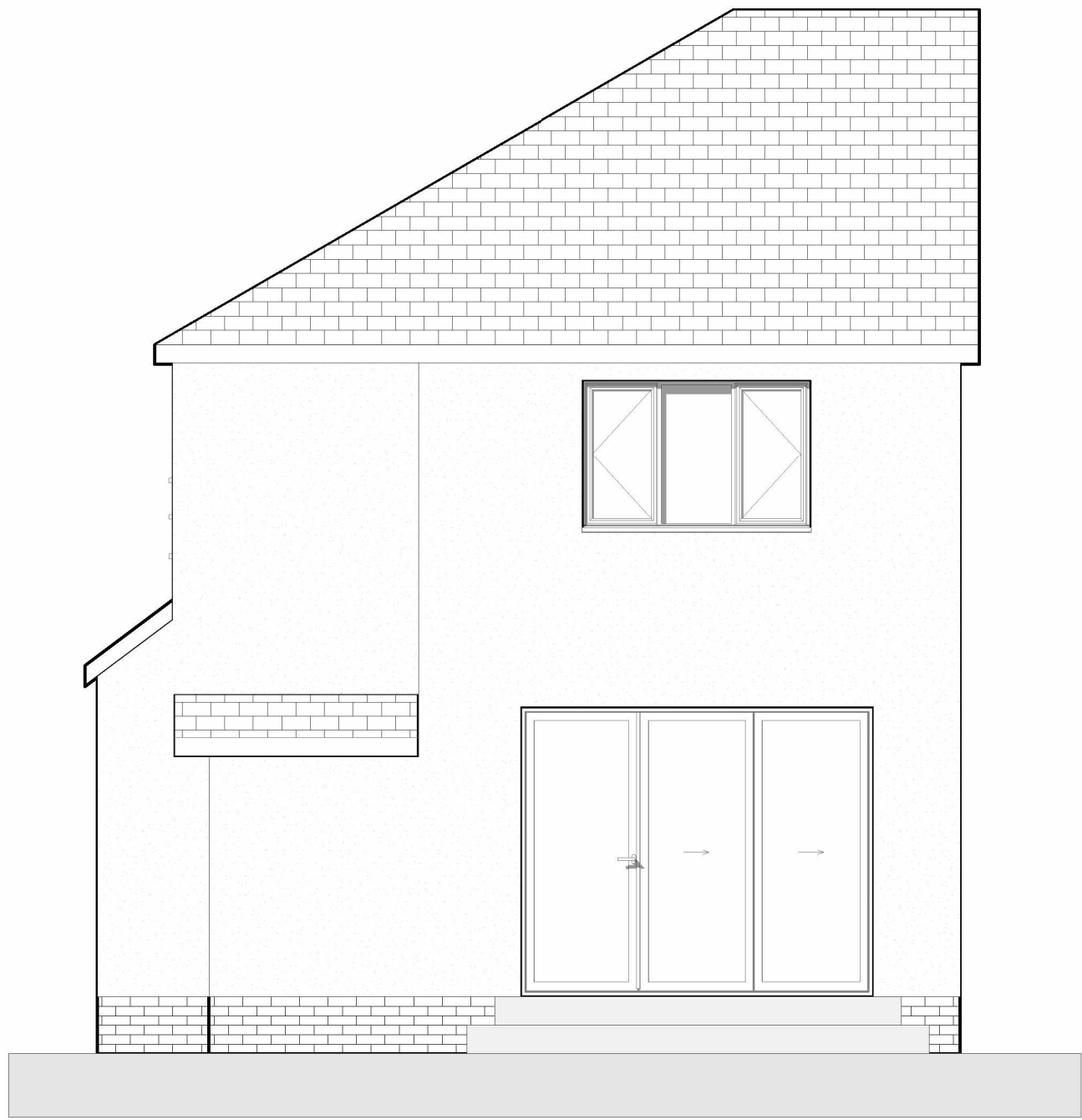
1 Existing Rear SCALE: 1 : 50
