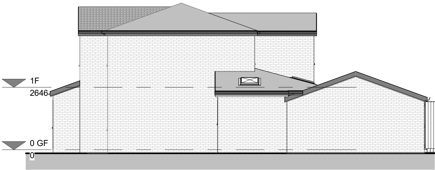
SIDE ELEVATION I 1:100
